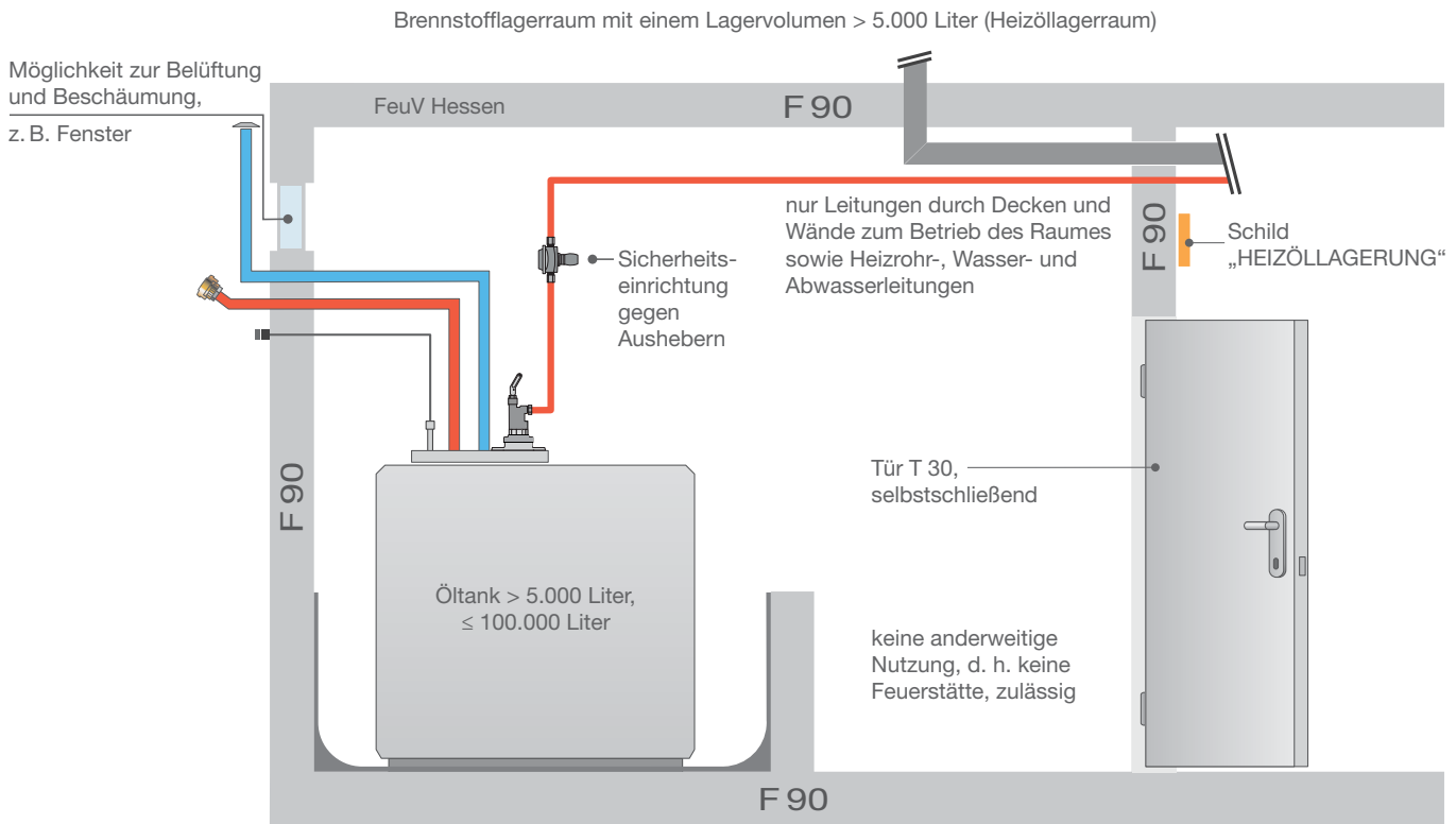
Grafik A 8-16 Anforderungen der FeuV Hessen an Heizöllagerräume
